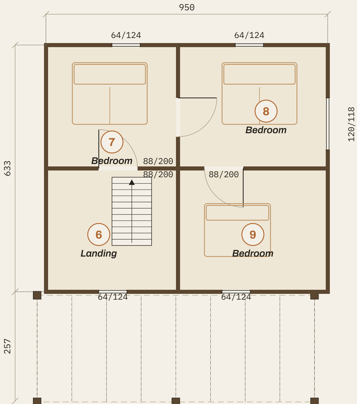
FIRST FLOOR · PIĘTRO
